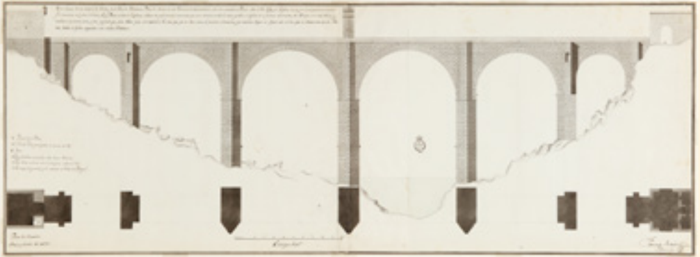
Dibujo del puente de Alcántara. Planta y alzado de la fachada de los tajamares. Fernando Rodríguez. Real Academia de Bellas Artes de San Fernando.
